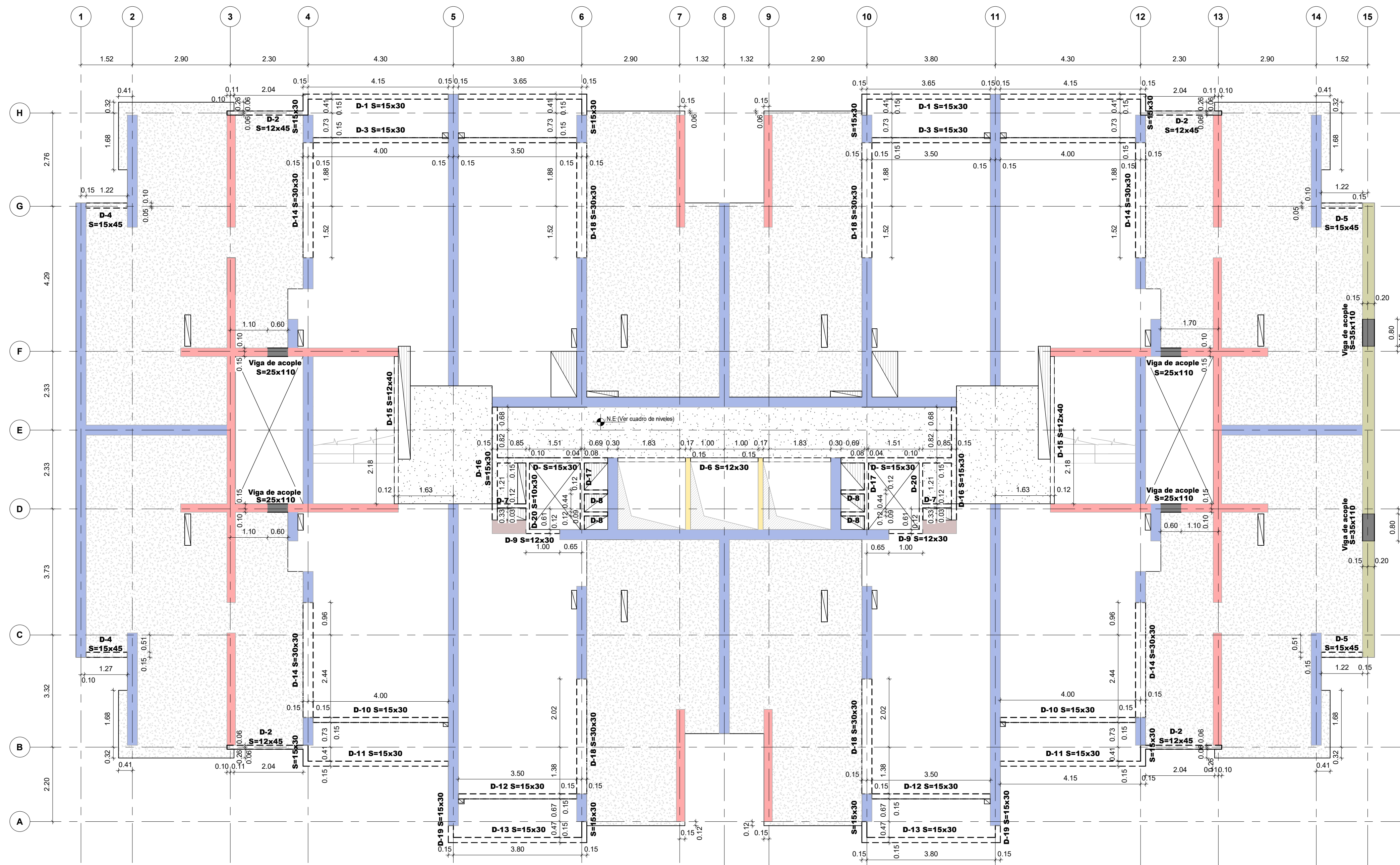
PLANTA LOCALIZACIÓN DE DINTELES PISO TIPO 2 ( PISO 16 A PISO 22 ) Escala 1 : 75
